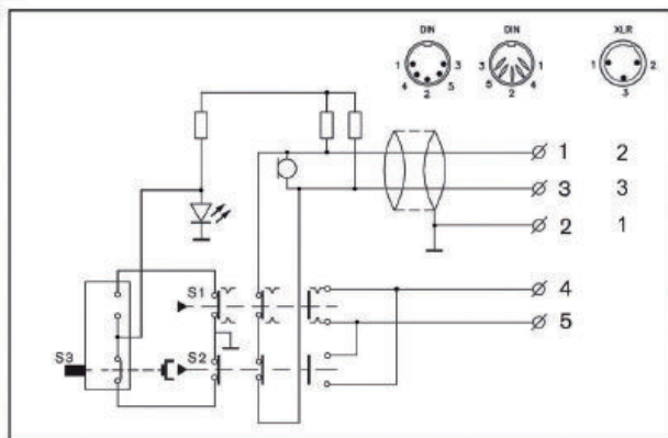
Kapcsolási rajz
