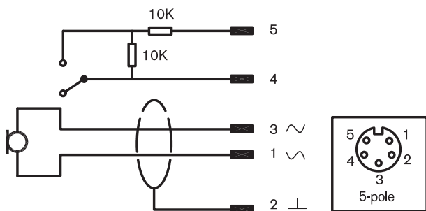
Kapcsolási rajz
