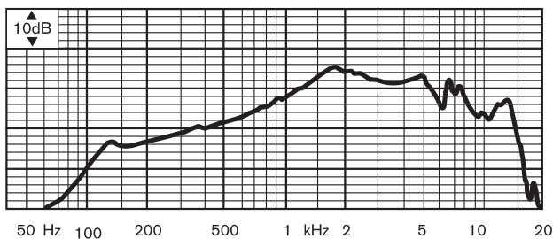
Frekvenciaátvitel
