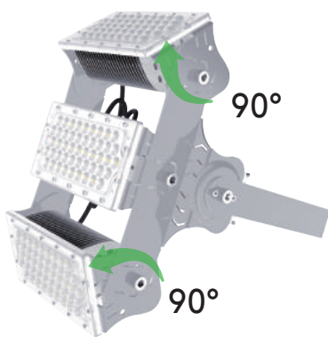
Rotatable Module
